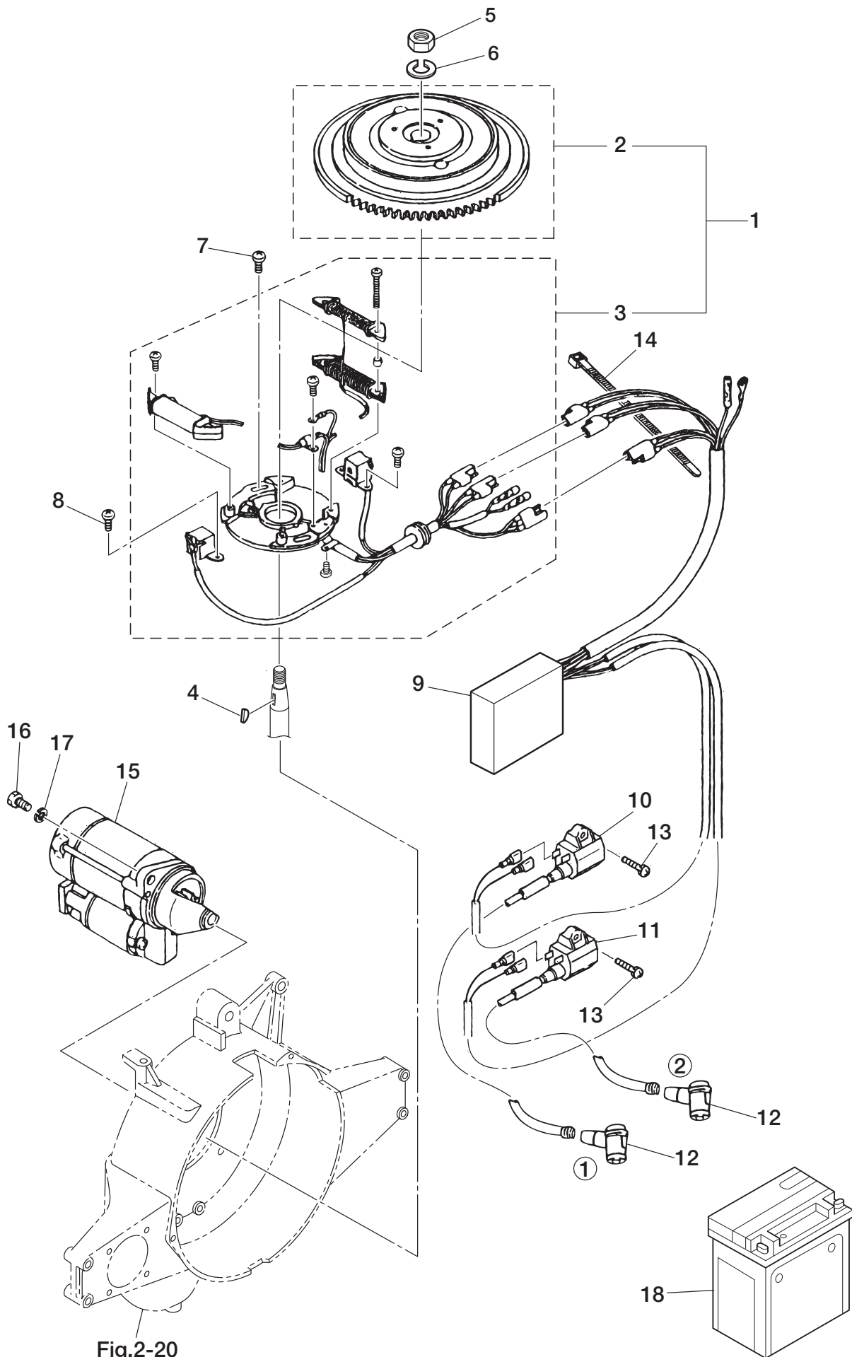
Fig. 9 MAGNETO
