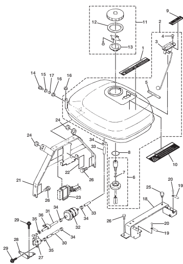
Fig. 22A FUEL TANK フュエルタンク (VC82ASE, VC82/85BS)
