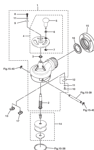
Fig. 16 DISCHARGE VALVE ディスチャージ バルブ
