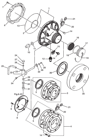
Fig. 15 DISCHARGE BALL VALVE ディスチャージ ボール バルブ
