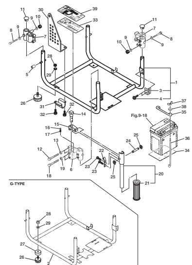
Fig. 18 FRAME フレーム
