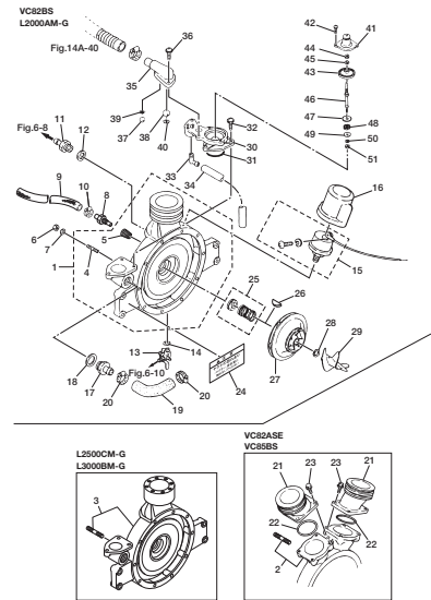
Fig. 14B VACUUM PUMP バキュームポンプ (VC82/85BS, G-TYPE)
