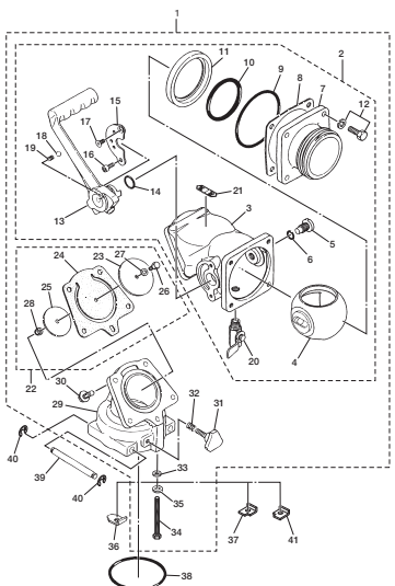
Fig. 15 DISCHARGE BALL VALVE ディスチャージ ボール バルブ
