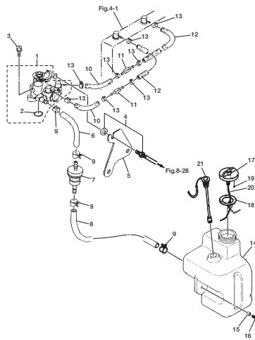
Fig. 14A VACUUM PUMP バキュームポンプ
